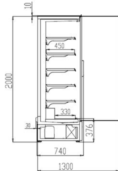
Coupe vitrine
